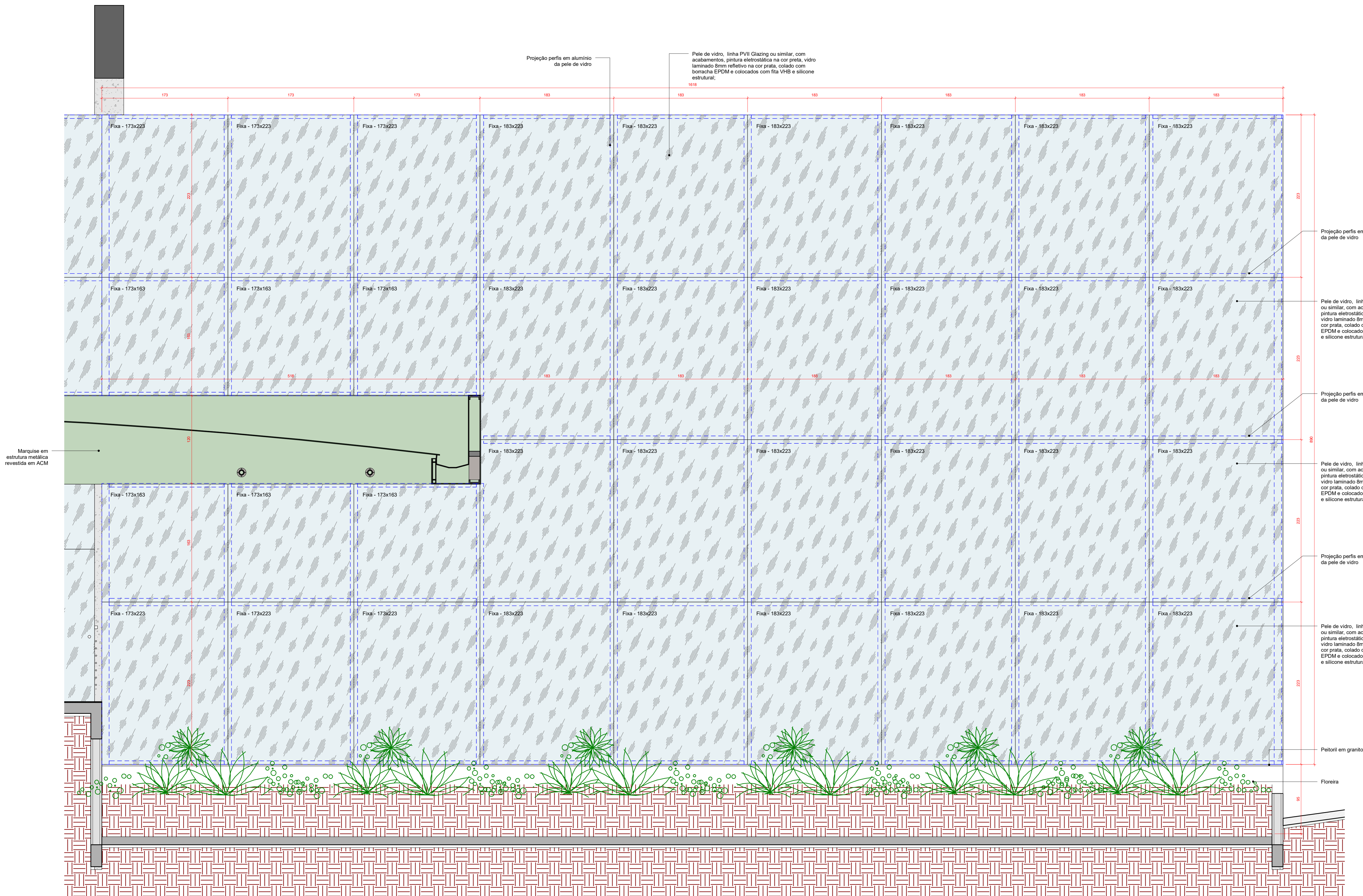
PELE DE VIDRO - VISTA C Escala 1 : 25
