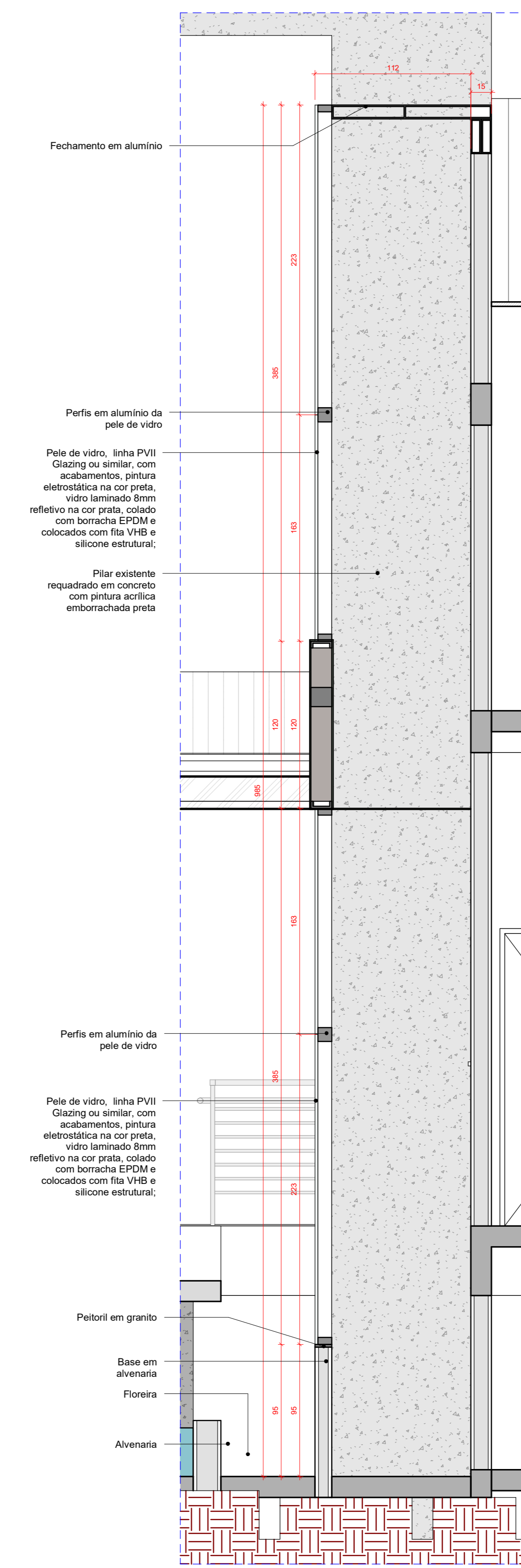
CORTE EE - PELE DE VIDRO Escala 1 : 25
