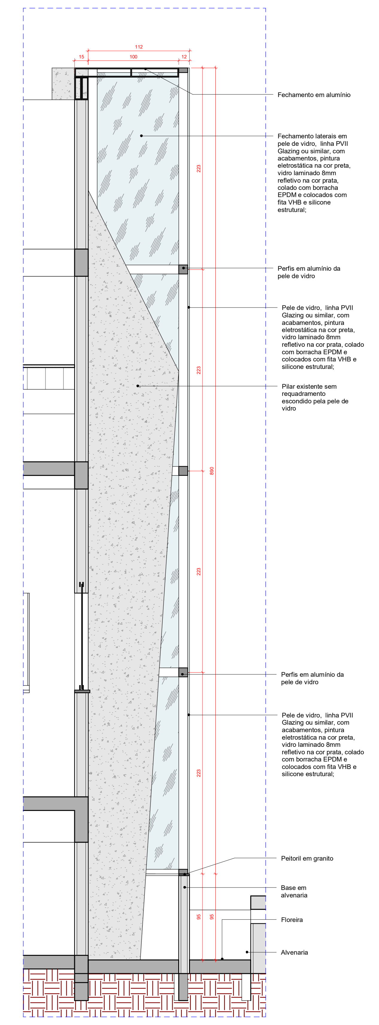
CORTE FF - PELE DE VIDRO Escala 1 : 25
